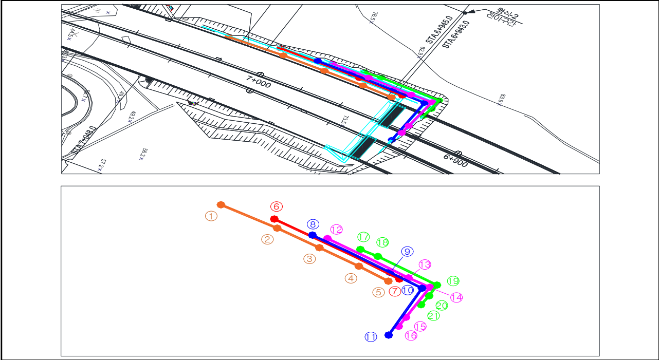
【그림 3.13】 계획선형 측량 현황
