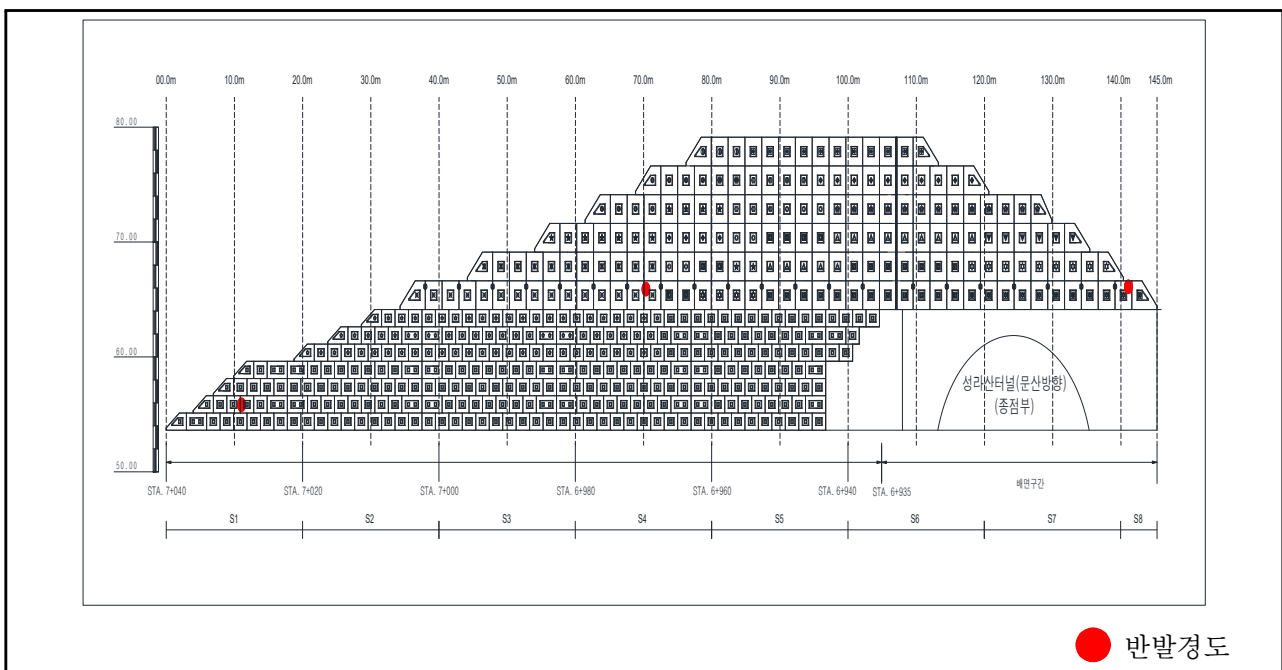
【그림 3.11】 재료시험 위치도
