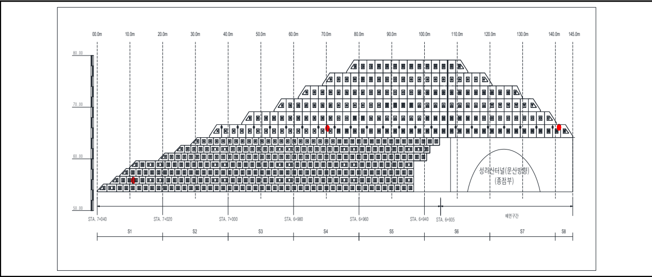
【그림 3.9】 옹벽 조사 분할구간
